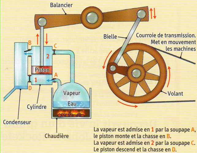
Machine à vapeur de James WATT - 1769
